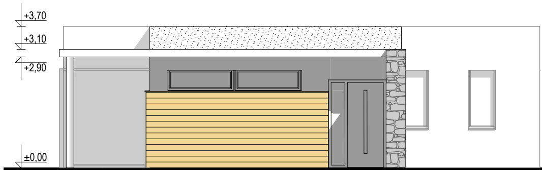
PROČELJE ISTOK
