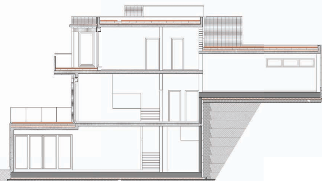
ZAPADNO presjek
