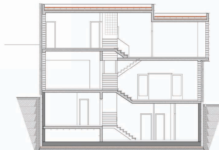
ISTOČNO presjek
