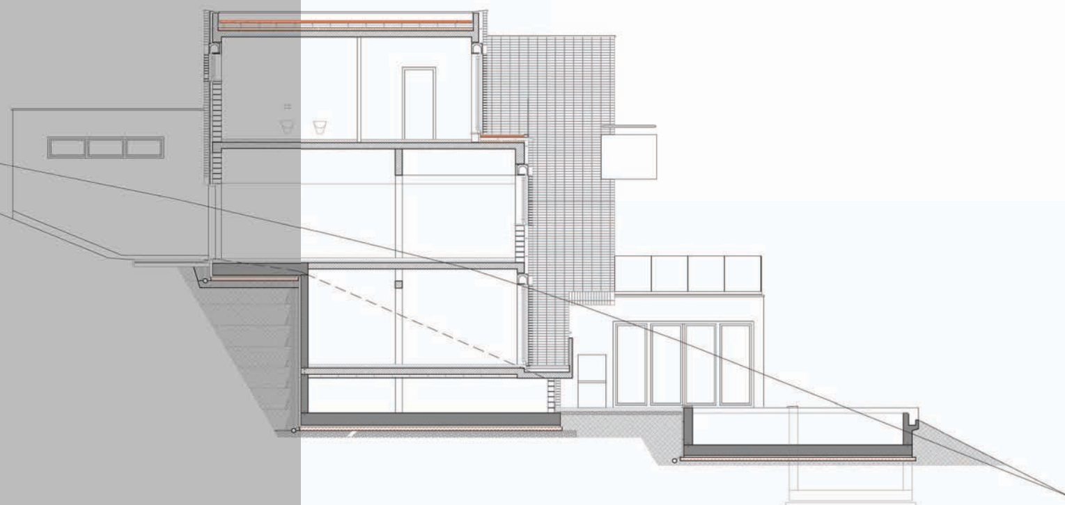
JUŽNO presjek
